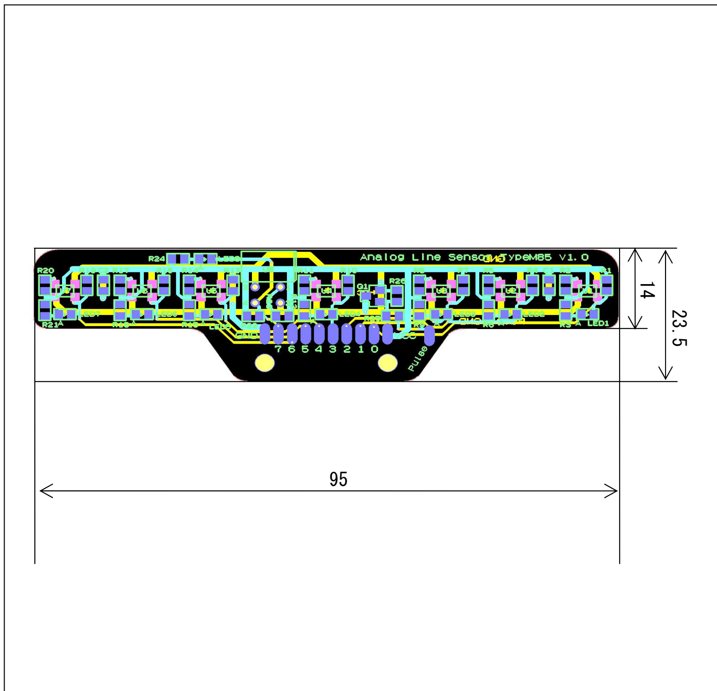
图 1 基板寸法图
